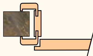
zárubeň v provedení folie nebo lamino (zaoblené hrany obložek)
