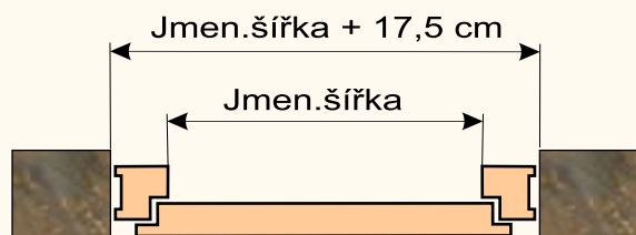
rámová zárubeň pro falcové dveře
