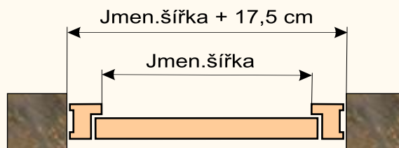
rámová zárubeň pro bezfalcové dveře
