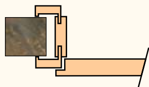
zárubeň pro dveře dýchované (ostré hrany obložek)
